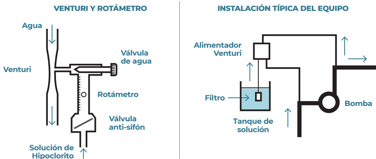
Ilustración. Esquema de un hipoclorador Tipo Venturi
