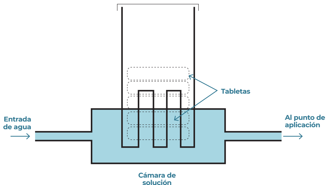
Ilustración. Hipoclorador a goteo
